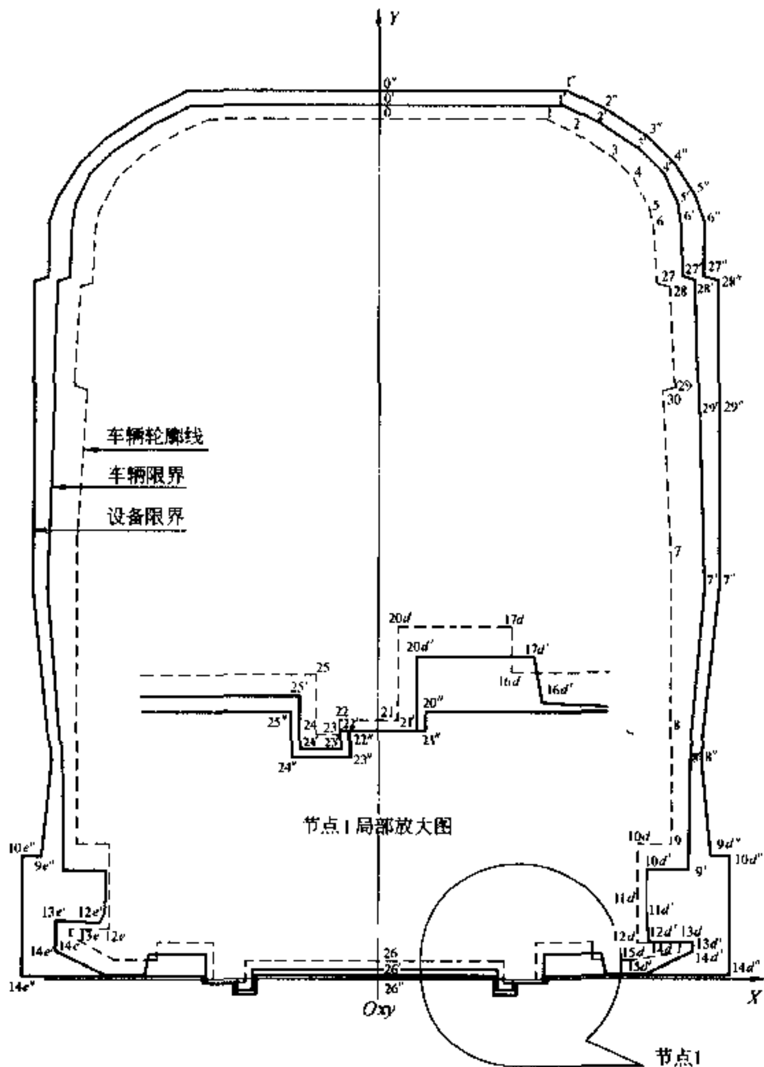
图 C.4 高架或地面直线地段车辆轮廓线、车辆限界、设备限界图
