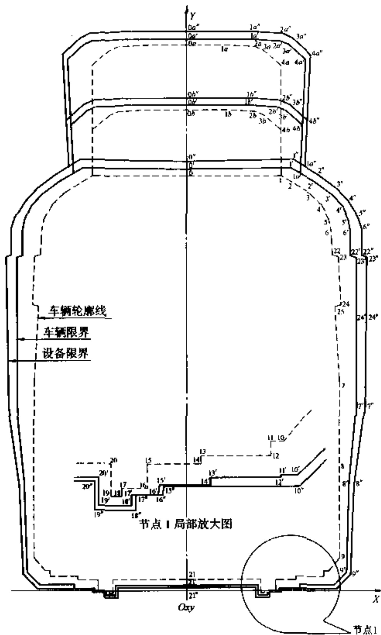
图 D.2 高架或地面直线地段车辆轮廓线、车辆限界、设备限界图
