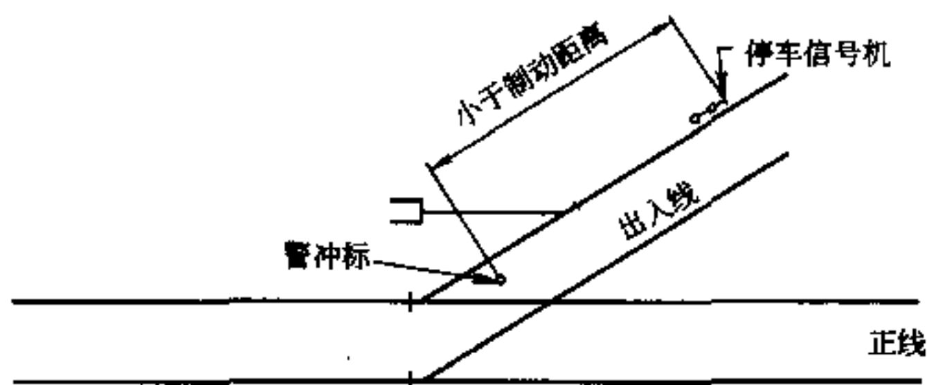
图1 出入线接正线形式
