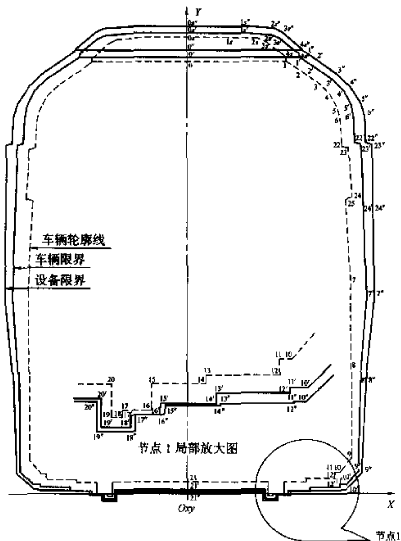
图 D.1 隧道内直线地段车辆轮廓线、车辆限界、设备限界图
