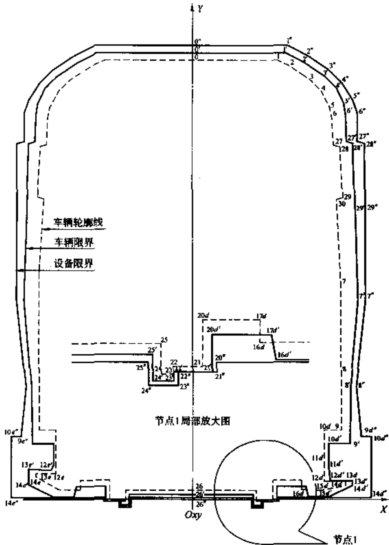
图 C.3 隧道内直线地段车辆轮廓线、车辆限界、设备限界图
