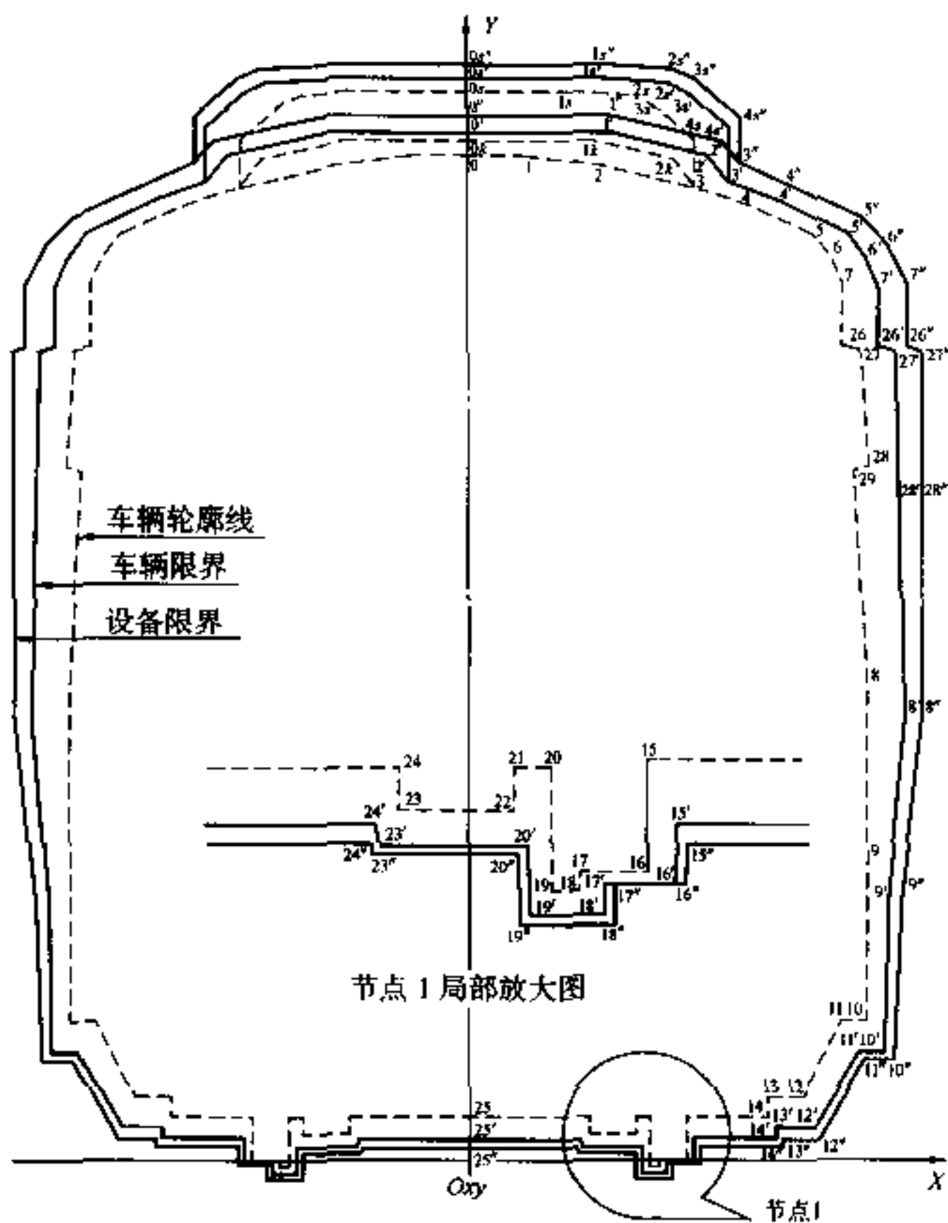
图 B.1 隧道内直线地段车辆轮廓线、车辆限界、设备限界图
