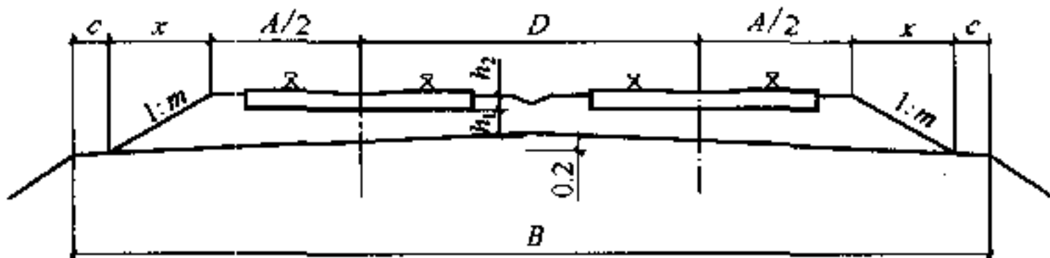
图5 双线非渗水土路基面示意
